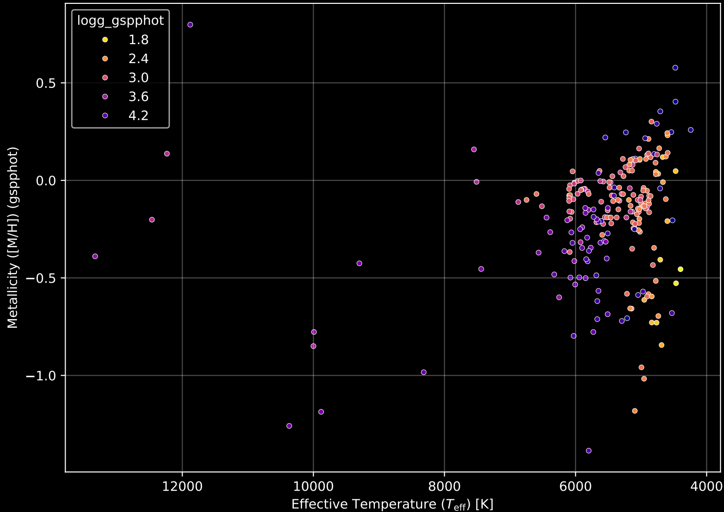
APOGEE DR17 Field: [205-03-C] Stellar Population Parameters (n= 227)
